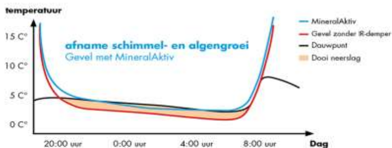
Voorbeeld van de relatie tussen temperatuur en dauw op de gevel - met MineralAktiv Gevelverf en conventionele gevelverf (gemeten op een koele septembernacht).
