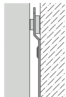
Wandbevestigingsset
