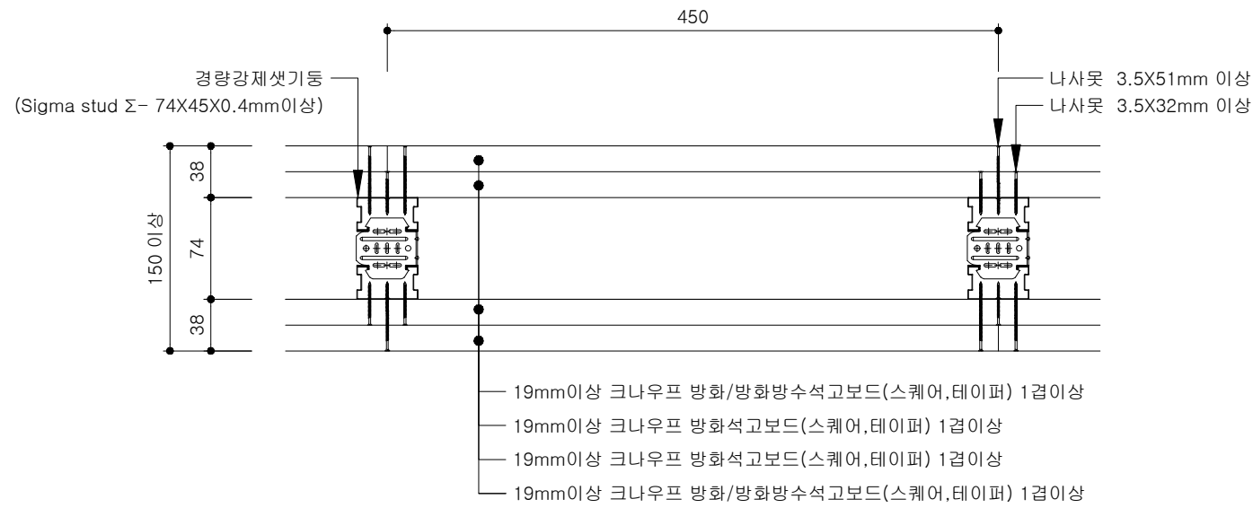
평면 상세도
