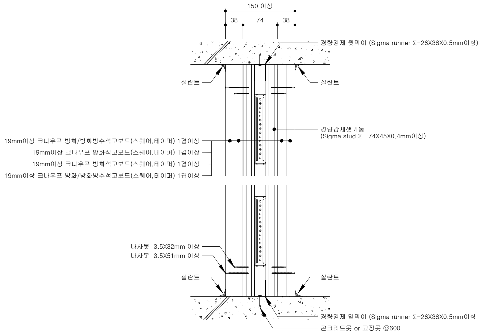
단면 상세도
