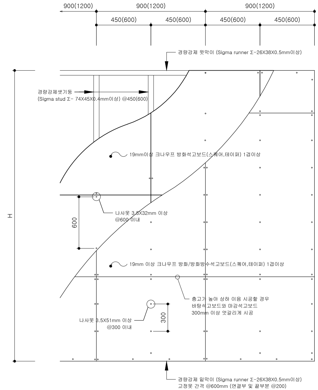
입면 상세도
