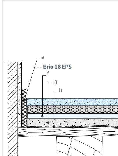
GB 2 Vægtilslutning
