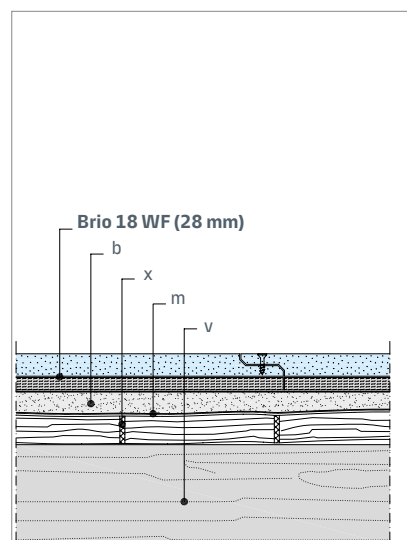
GB 9 Træbjælkelag
