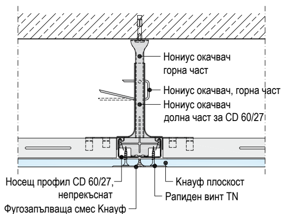
D113.bg –B5 Надлъжен ръб - едно ниво/Нониус окачвач
