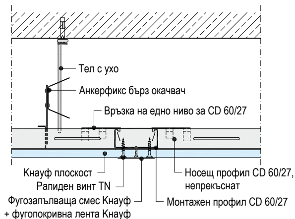
D113.bg –C1 Челен ръб - едно ниво/анкерфикс
