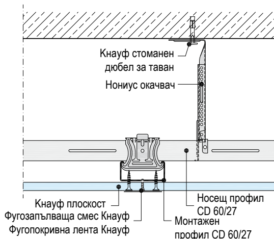
D112.bg –C4 Челен ръб – Носещ профил/монтажен профил/анкерфикс
