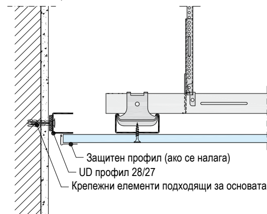
D112.bg – D7 Плъзгаща връзка към стена
