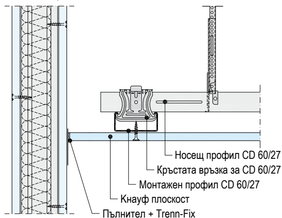
D112.bg –D6 Плъзгаща връзка към стена
