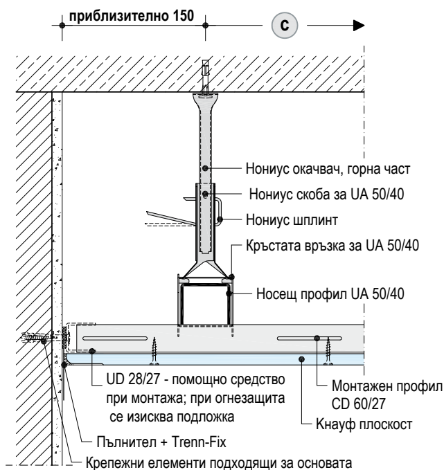
D116.bg –B1 Надлъжен ръб - носещ профил/монтажен профил/нониус скоба
