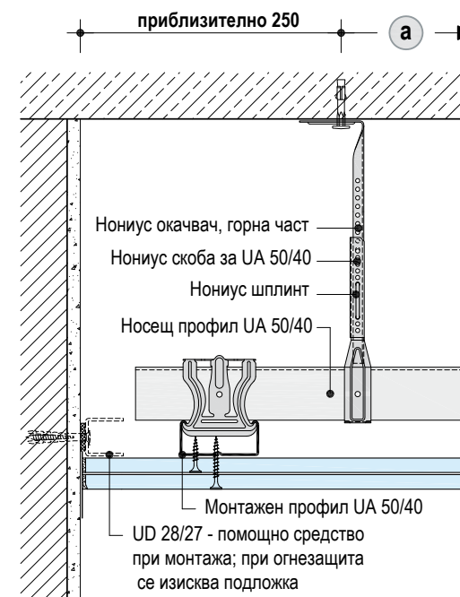
D116.bg –D1 Връзка към стена
