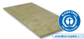
Trittschall-Dämmplatte TPE (Nutzlast ≤ 10 kPa)
