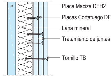
W633.es-VM1 Junta horizontal
