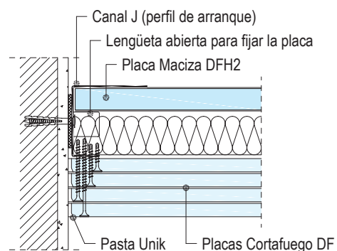
W636.es-A1 Encuentro con muro
