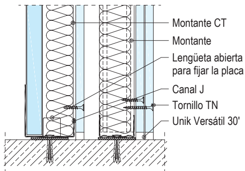
W634.es-VU1 Encuentro con forjado inferior
