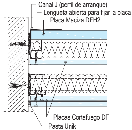
W634.es-VM1 Junta horizontal
