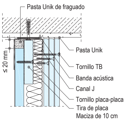
W633.es-VO1 Encuentro con forjado superior
