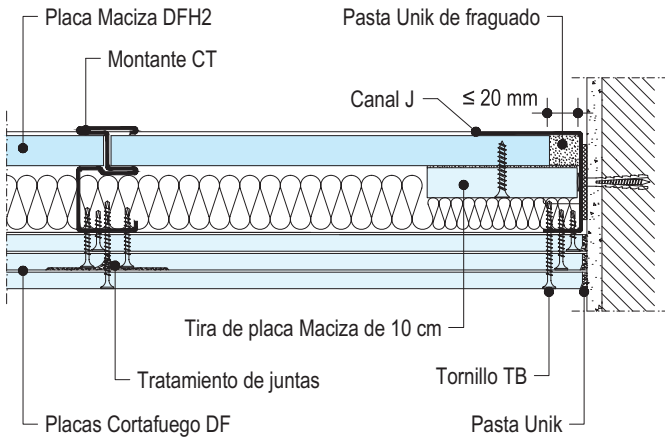
W634.es-VO2 Encuentro flotante
