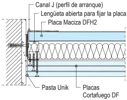
W633.es-VU1 Encuentro con forjado inferior
