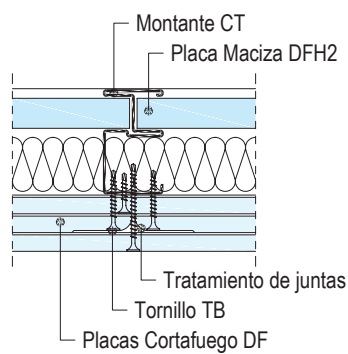
W633.es-B1 Junta vertical
