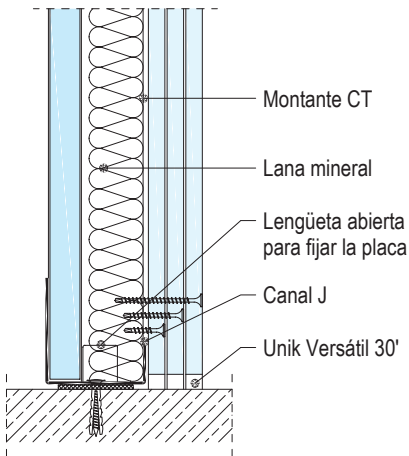
W633.es-VU1 Encuentro con forjado inferior
