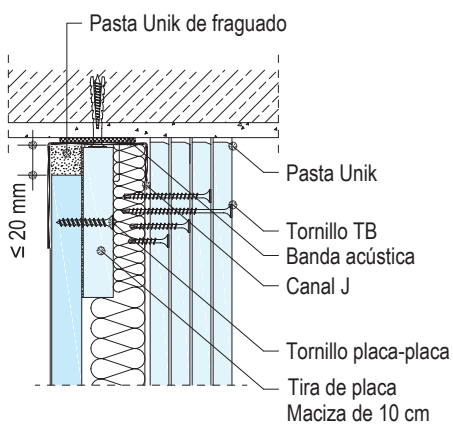
W636.es-VO1 Encuentro con forjado superior
