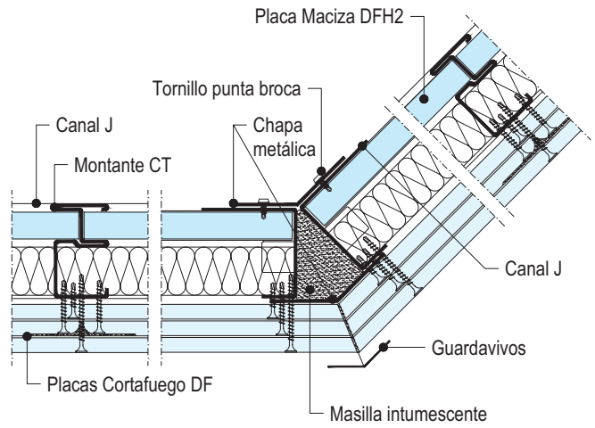
W633.es-VO2-H1 Encuentro flotante
