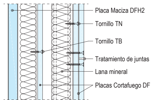
W634.es-VM1 Junta horizontal
