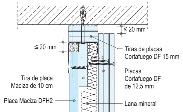
W633.es-BFU1 Junta de dilatación
