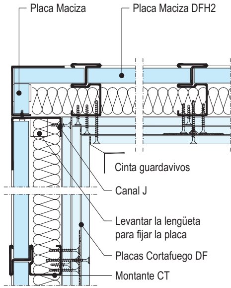
W633.es-B2 Fijación de la última placa Maciza
