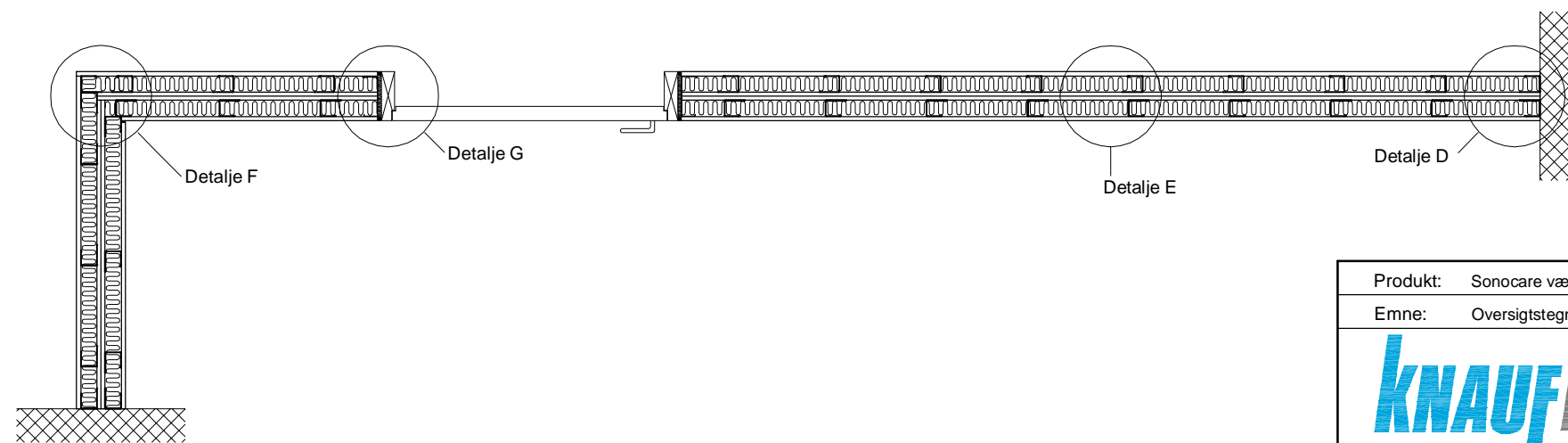
Snit B-B
