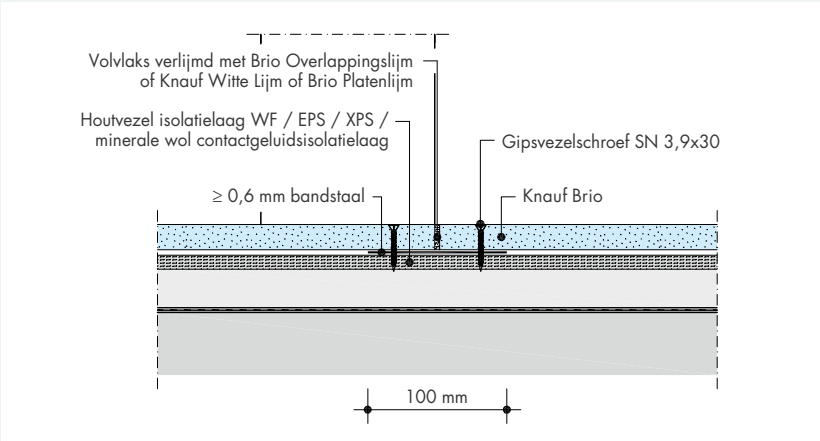
Detail 5: Doorsnede A-A bij uitvoering met bandstaal
