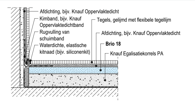
Detail 7: wandaansluiting in vochtige ruimtes
