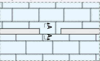
Montage zonder passtuk, met stompe naad
