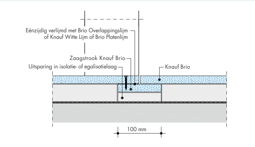
Detail 4: doorsnede A-A bij uitvoering als dilatatievoeg
