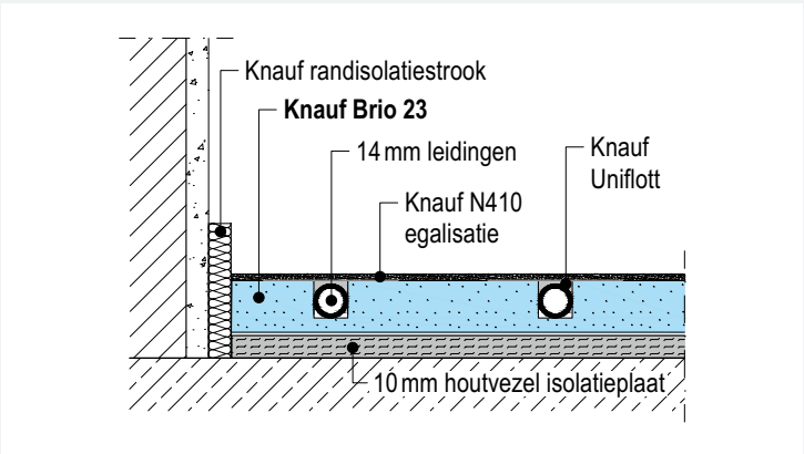
Detail 2: principe van Knauf Brio met ingefreesde vloerverwarming
