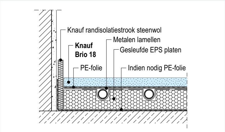
Detail 1: principe van Knauf Brio op vloerverwarming
