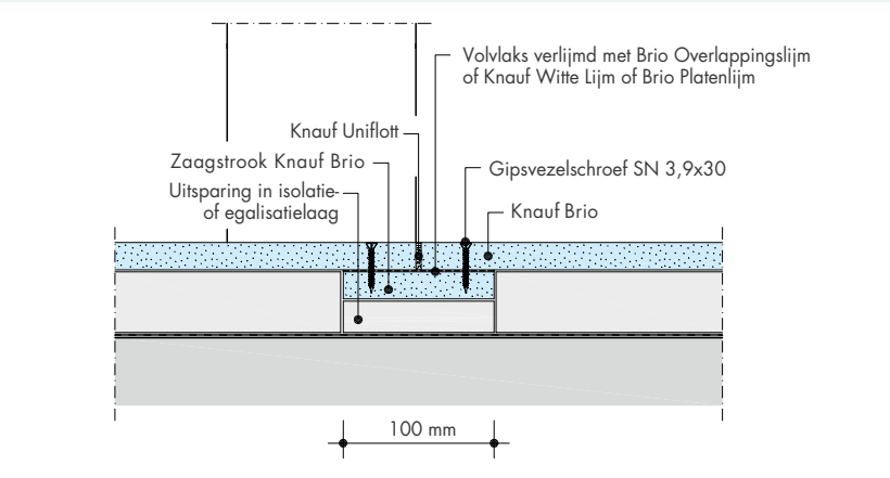
Detail 3: doorsnede A-A bij uitvoering met plaatstrook
