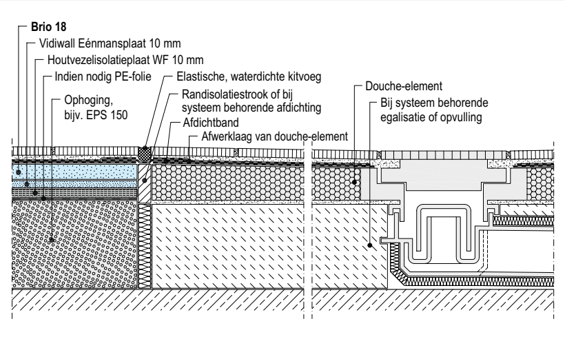
Detail 8: vloeraansluiting op douche-element zonder drempel
