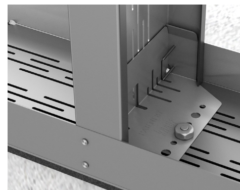
Nail Impact fastør skinne, stolpe og Nail Bracket. 2 stk. Nail Impact pr. side og 4 stk i alt.
