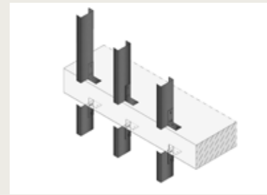
2. Install exterior stud frame
