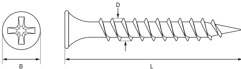
Tegning af SN 3,5 skrue til visualisering af mål i tabellen Produktdata
