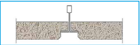
BORD E (SK-06-)
