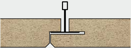
DALLE À BORDS OSSATURES CACHÉES Type de bords : VK-10 (D) Profilé : T35
