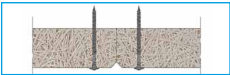
Pose FMV (AK-01) avec vis Organic
