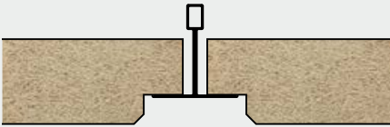
DALLE À BORDS SEMIENCASTRÉS - T35 Type de bord : SK-06 T35 [E] Profilé : T35
