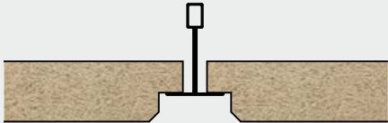
DALLE À BORDS SEMIENCASTRÉS - T24 Type de bord : SK-06 T24 [E] Profilé : T24
