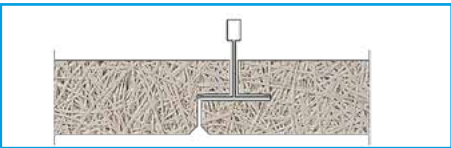
BORD D (VK-10) (uniquement T-35) Biseauté à ossature cachée démontable
