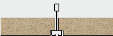
DALLE ENCASTRÉE OSSATURE SILHOUETTE Profilé : T15 Silhouette
