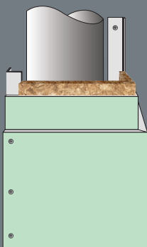
כיסוי אקוסטי כפול מוכן בצורת (L) לחיפוי צנרת אינסטלציה
