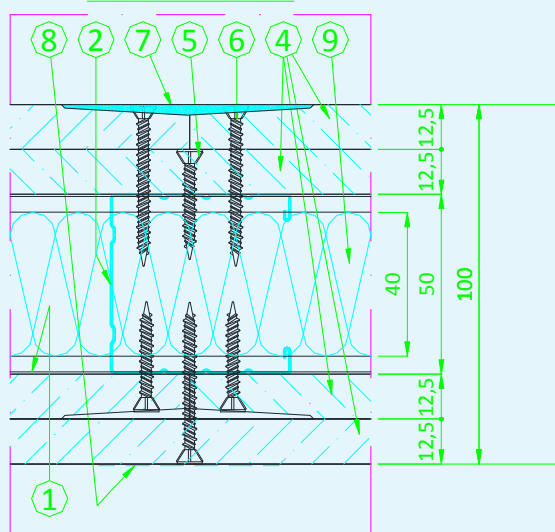
Particolare "D"
