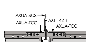
AXT-T42-Y Transizione lastre metalliche / lastre metalliche
