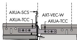
AXT-VEC-W Transizione cartongesso / lastre Vector
