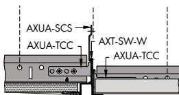
AXT-SW-W Transizione cartongesso / lastre lay-in
