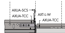
AXT-L-W Transizione cartongesso / lastre lay-in
