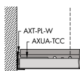
AXT-PL-W Dettaglio perimetrale per lastre lay-in
