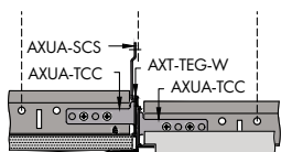
AXT-TEG-W Transizione cartongesso / lastre Tegular
