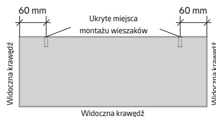
Dwuwarstwowy panel Baffe z powierzchnią HERADESIGN® i ukrytymi elementami mocującymi do montażu wieszaków
