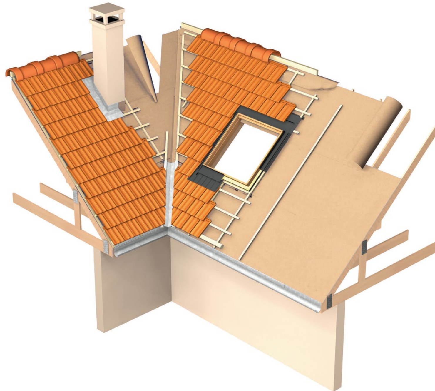
4 Plaatsingsprincipe van een onderdakscherm
