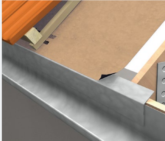
1 Aansluiting op de dakgoot
