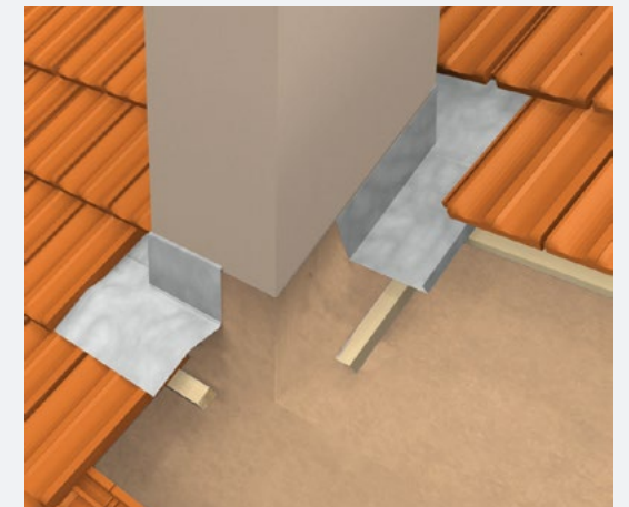
6 Aansluiting op een schoorsteen
