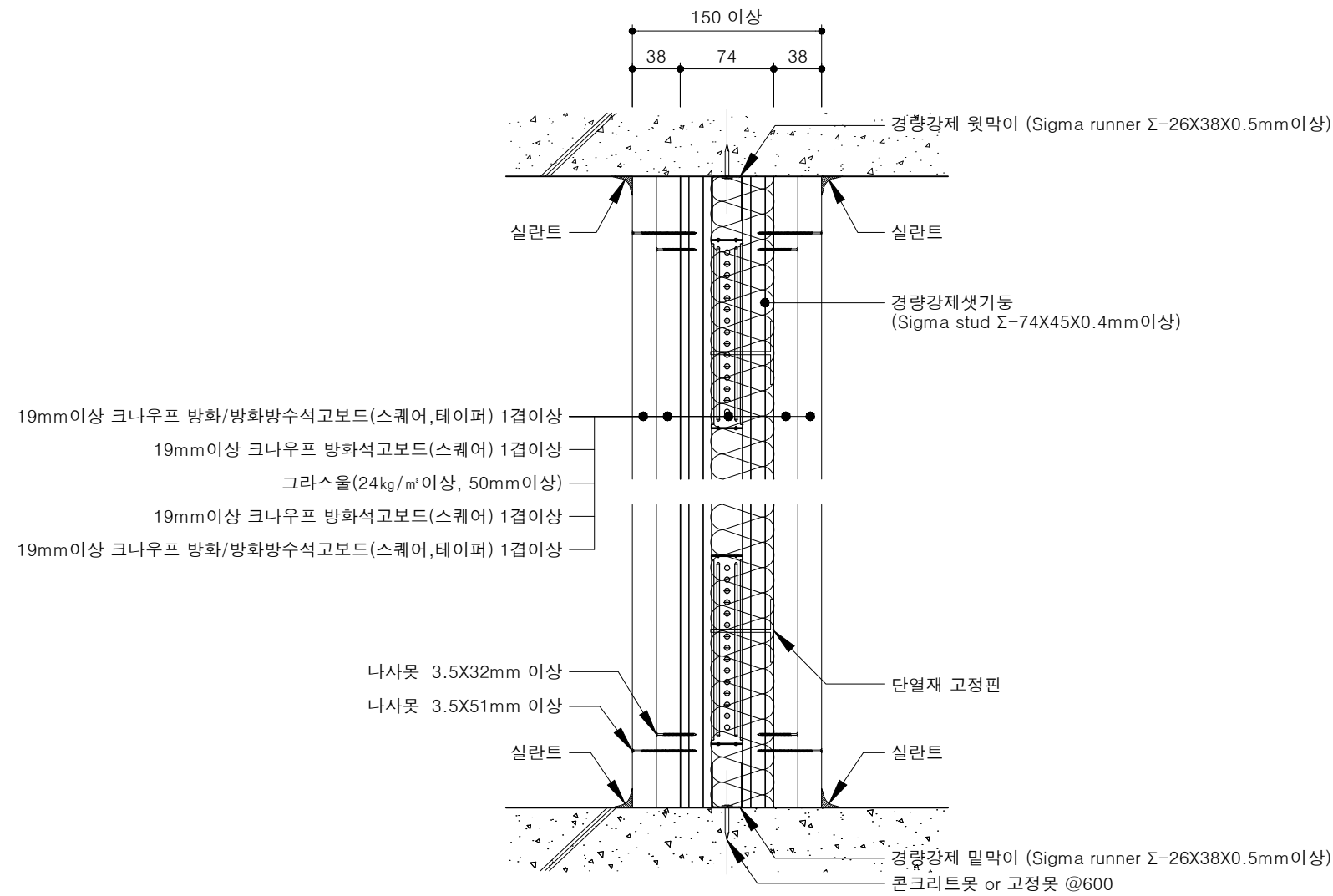
단면 상세도
