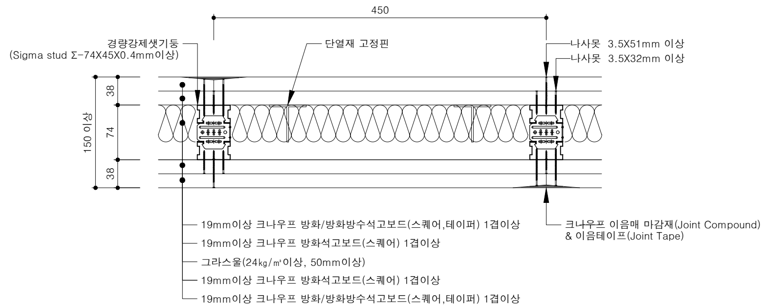
평면 상세도
