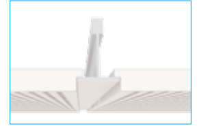
E+-reuna [E+] (TEGULAR) / T15 TAI T24 Upotettu kehikko Malleille Unity 3, Unity 4, Unity 9 ja U 8|15|20
