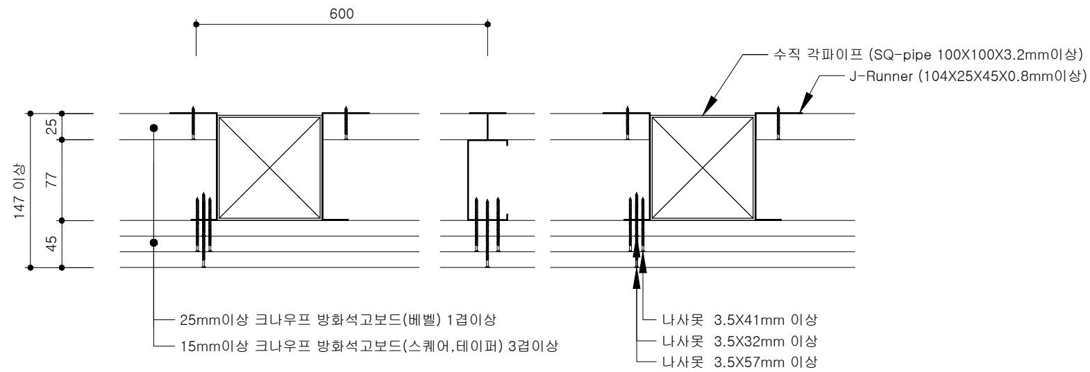
평면 상세도
