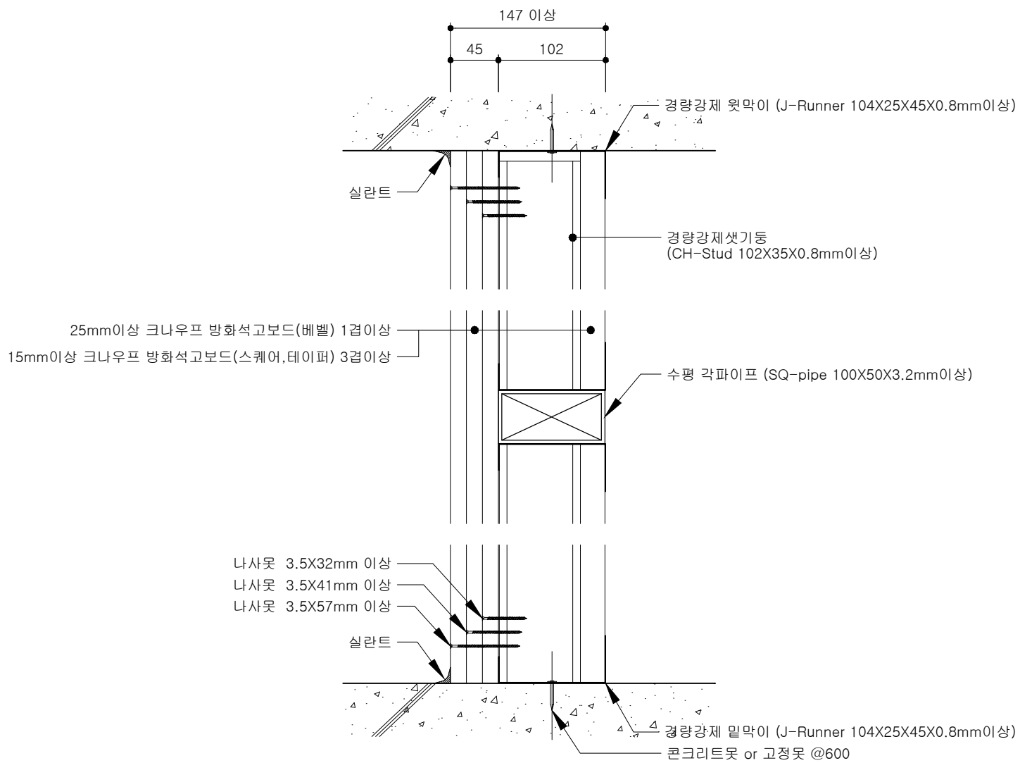
단면 상세도
