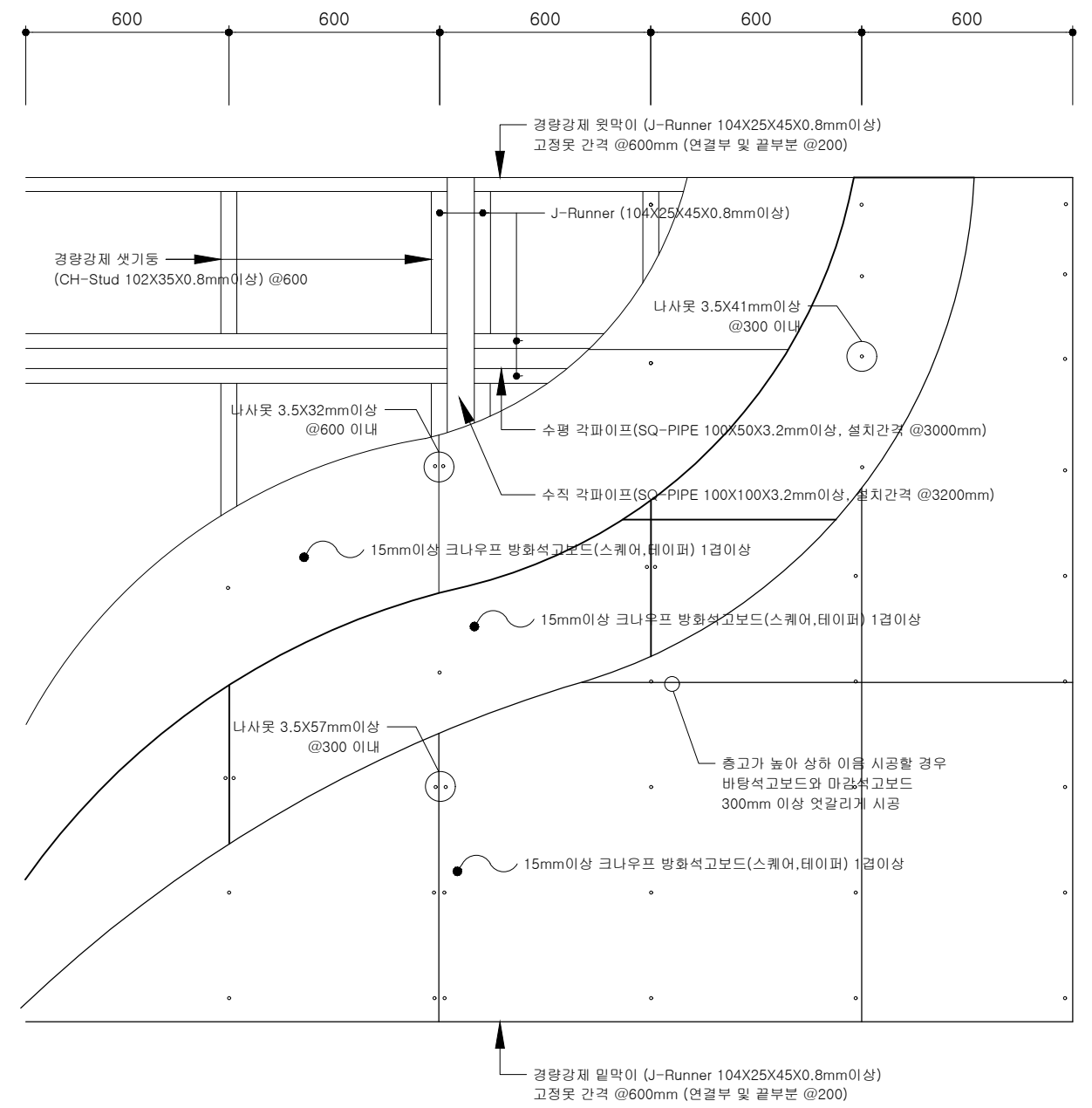
입면 상세도
