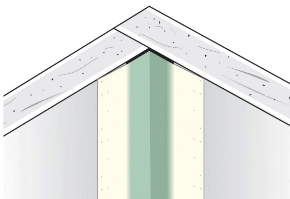
Illustration af hjørneprofilets placering på et indvendigt hjørne.
