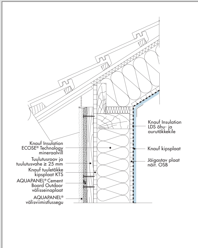
W681-DA-V1 Liitumine kaldkatusega, lahendus 1
