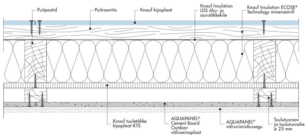
W681-H1 Horisontaallõige, lahendus 1
