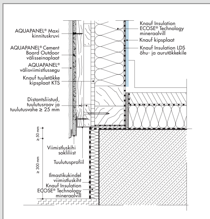
W681-SO-V1 Liitumine põrandaplaadiga
