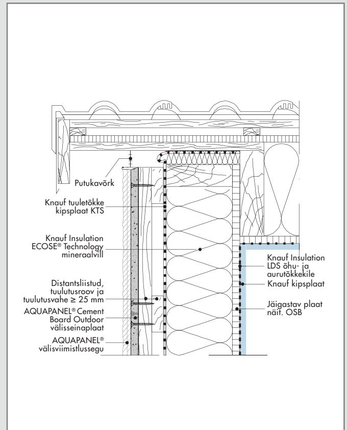
W681-DA-V2 Liitumine kaldkatusega, lahendus 2
