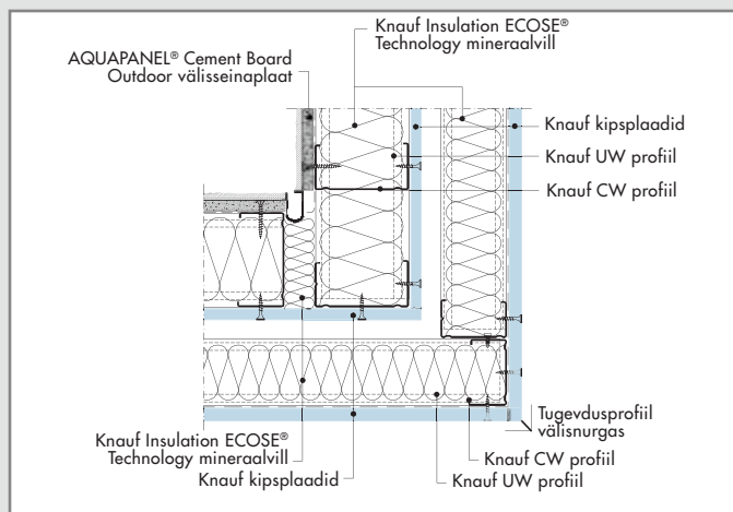
W387E-DBFU1 Sisenuurk paisumisvuugiga
