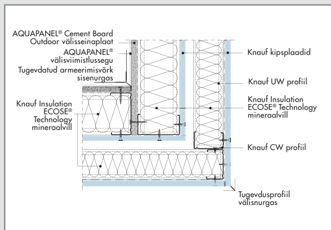
E387E-D1 Sisenuurk paisumisvuugiga
