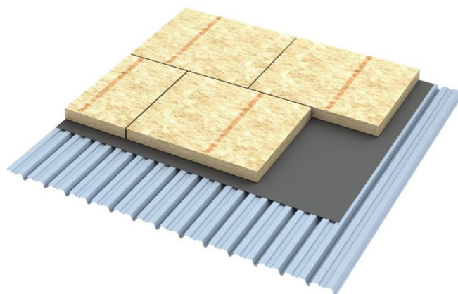
Fig. 1 – Principe de pose sur tôles d'acier profilées avant fixation
