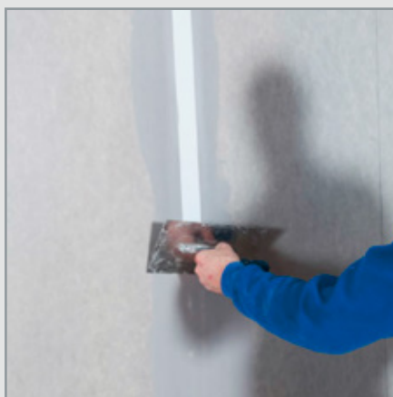
Krok 4: Přetmelte pásku systémovým tmelem Drystar-Filler.
