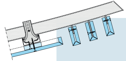
Πλάγιο τμήμα οροφής με λοξές λωρίδες
