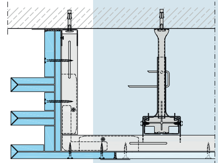
Κλιμακωτή οροφή με οριζόντιες λωρίδες
