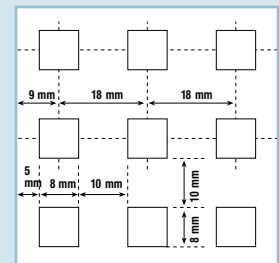
Διάτρητη γυψοσανίδα Κнауφ 8/18Q
