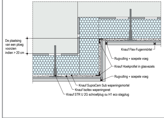
P329.be-FU-H4 Dilatatievoeg
