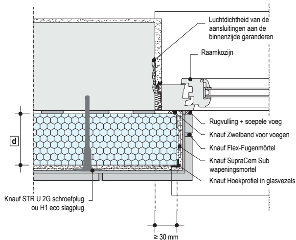
P329.be-FE-H2 Kozijn gelijk met het metselvlak
