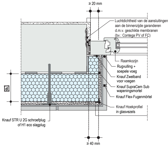
P329.be-FE-H1 Kozijn terruggliggend op het metselvlak
