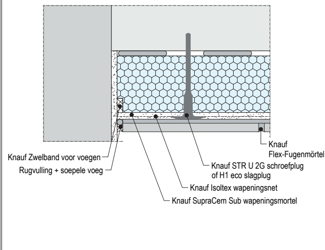
P329.be-FU-V1 Joint de fractionnement horizontal
