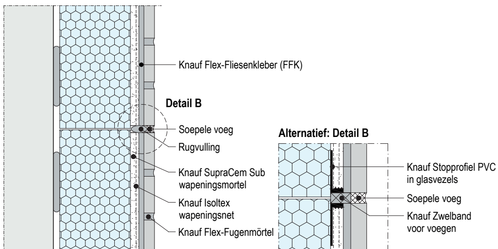
P329.be-FU-V1 Joint de fractionnement horizontal
