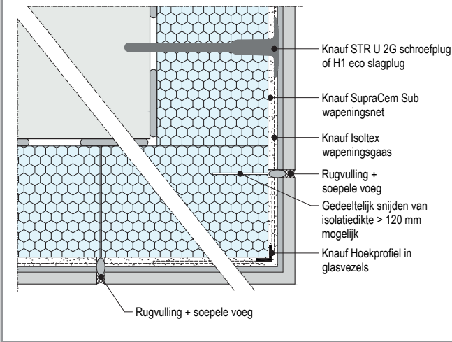
P329.be-FU-H3 Aansluiting met een bestaand bouwelement
