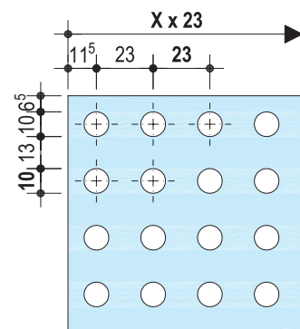
Perforación Redonda 10/23 R
