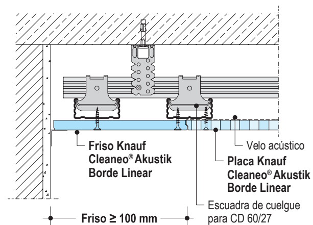
D127.es-D4 Encuentro con muro - Friso no plastecido
