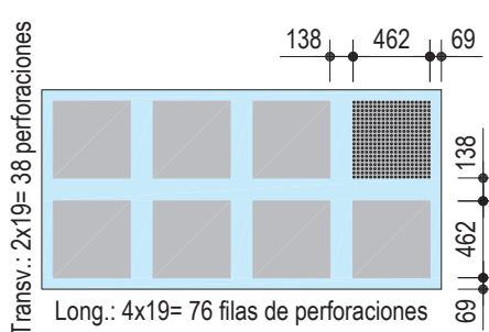
Diseño B5 – 12/25 R o 12/25 Q
