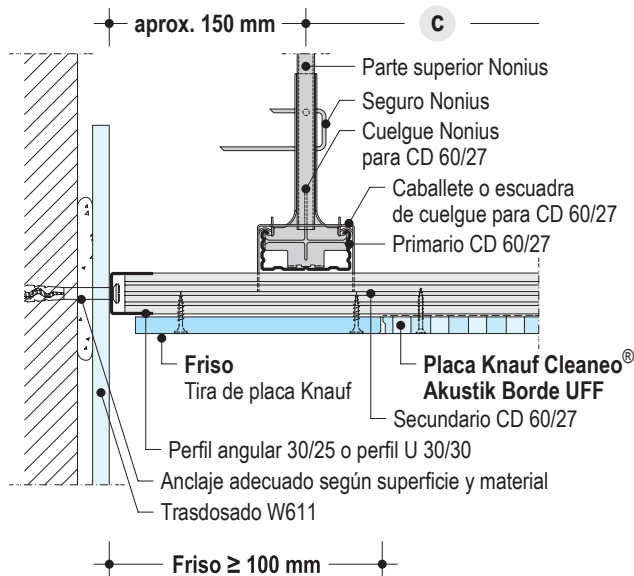
D127.es-A1 Encuentro con muro - Junta vista
