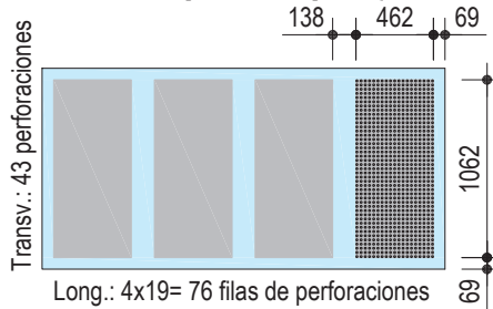
Diseño B6 – 12/25 R o 12/25 Q
