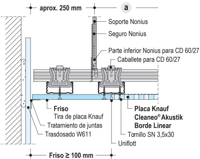
D127.es-D3 Encuentro con muro - Friso plastecido
