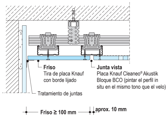
D127.es-D2 Encuentro con muro - Friso con junta vista
