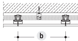
Modulación Secundarios
