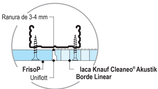
▪ Encuentro de friso con placa Cleaneo® Akustik - Borde Linear
