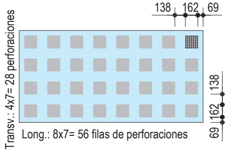
Diseño B6 – 12/25 R o 12/25 Q
