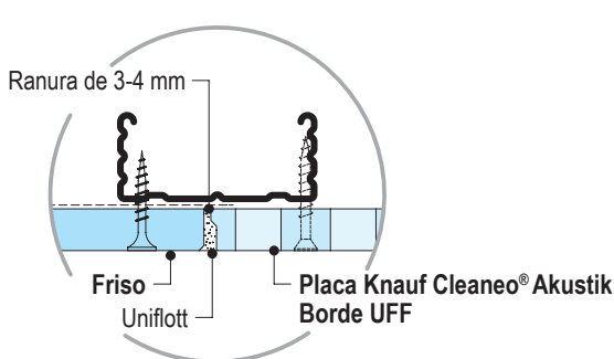
▪ Encuentro de friso con placa Cleaneo® Akustik - Borde UFF
