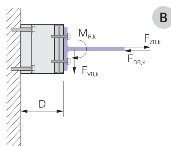
Horizontale montage (B)
