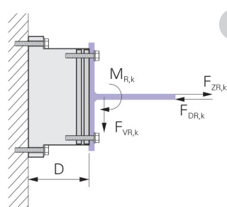
Vertikale montage (A)
