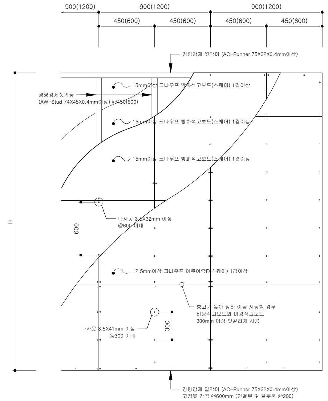
입면 상세도
