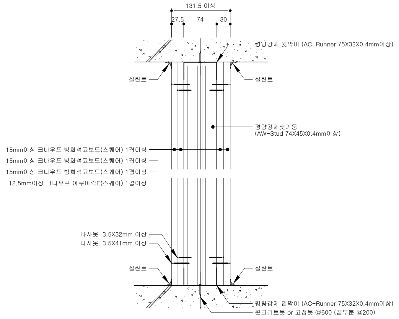
단면 상세도
