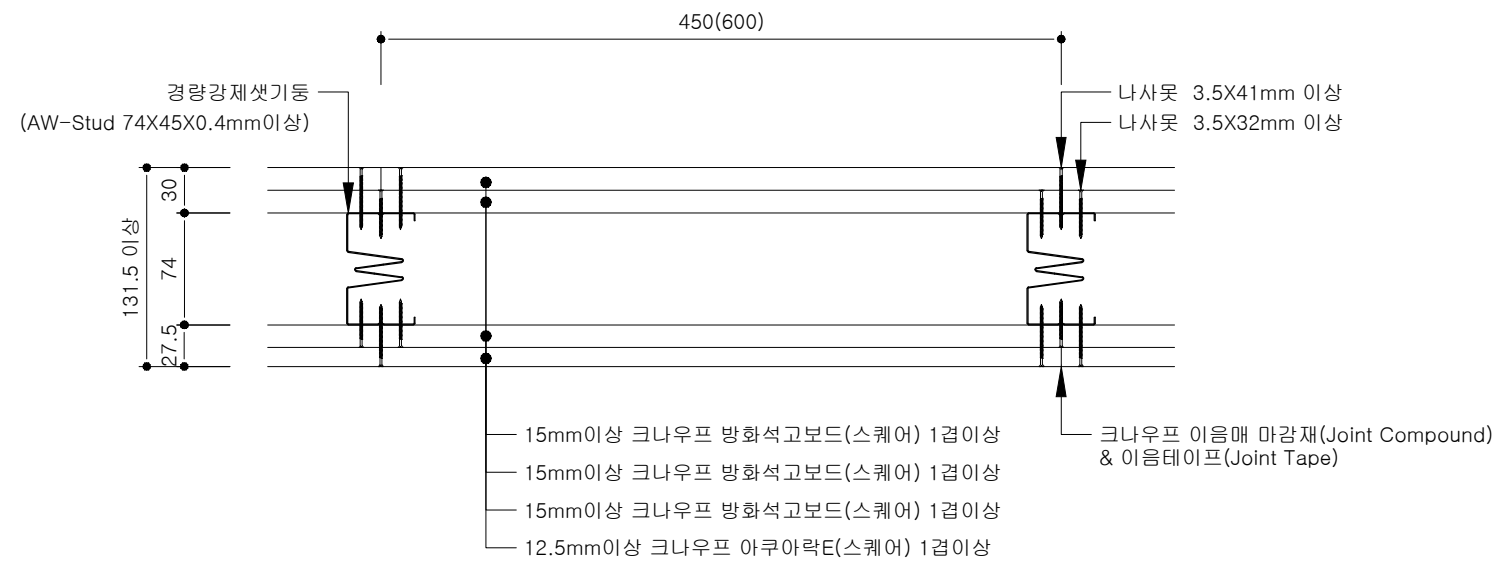
평면 상세도
