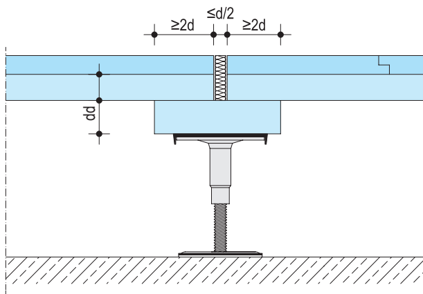
F182.es-V41 Suelo técnico Tecnosol Plus 25+18 Junta de control con protección al fuego
