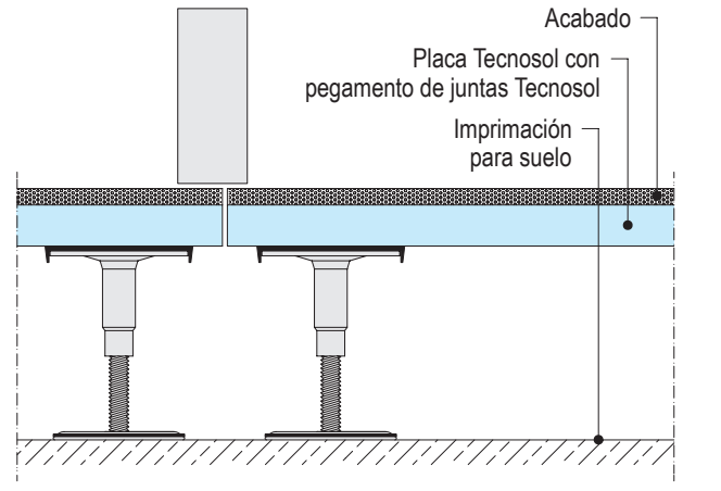
F181.es-V11 Junta de control con protección al fuego
