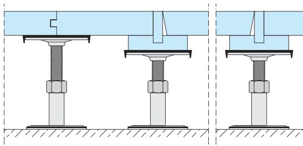
F181.es-V13 / F181.es-V14 Ejemplos: Travesaños de refuerzo
