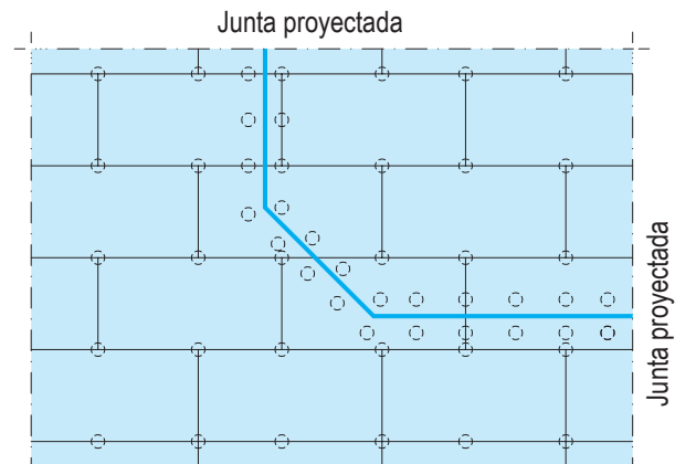
Junta acústica para separar dos ambientes proyectados sin transmisión de ruido de impacto
