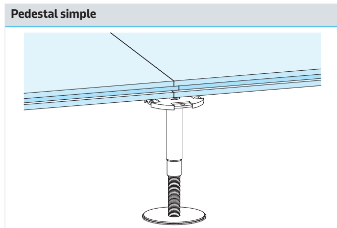
Pedestal simple M12 para placa Tecnosol
