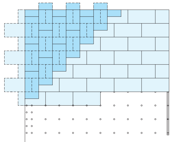
Desplazamiento óptimo de las juntas a 30 cm
