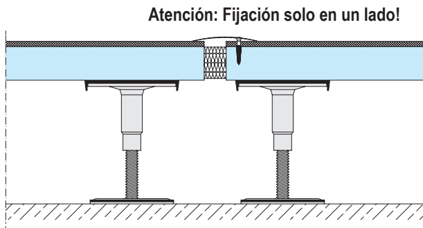
F181.es-V15 Ejemplo: Instalación de un tapa juntas
