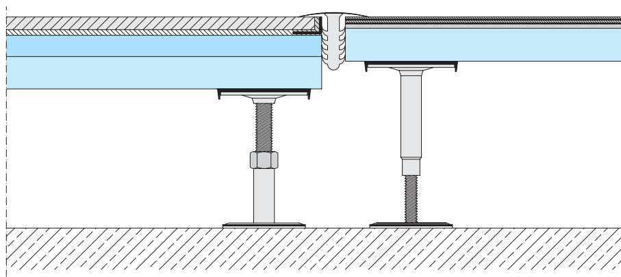
F182.es-V36 Cambio de sistema de F182.es a F181.es (por ej. en la zona de la puerta)
