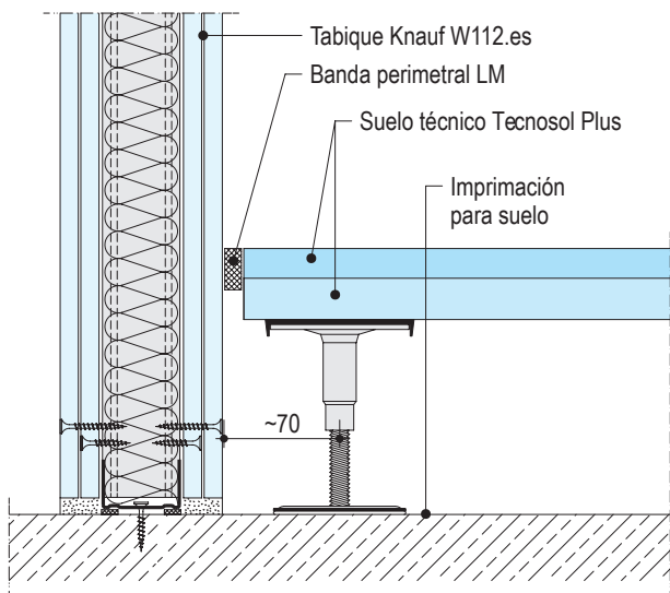
F182.es-V31 Tecnosol Plus 25+18
