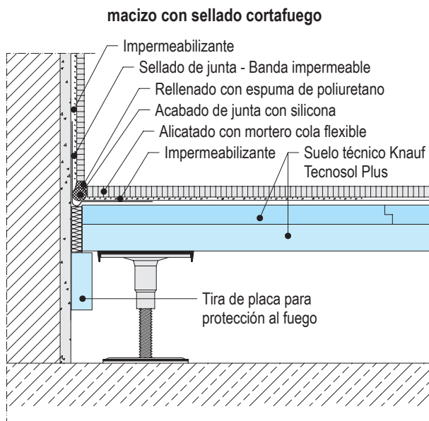
F182.es-V39 Tecnosol Plus 32+18 Barrera cortafuego
