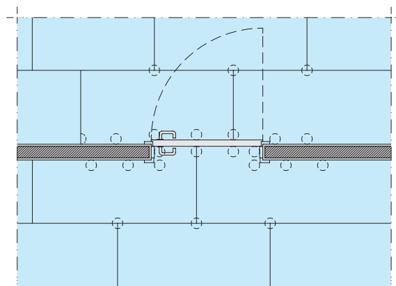
En las zonas de aberturas de puertas, reforzar la junta con pedestales
