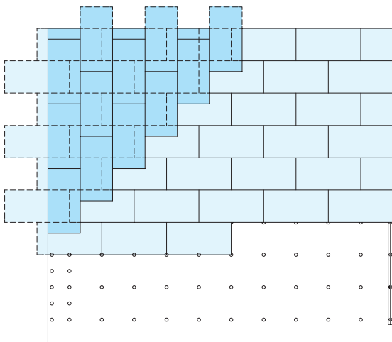
Desplazar las juntas de la segunda capa al menos 20 cm
