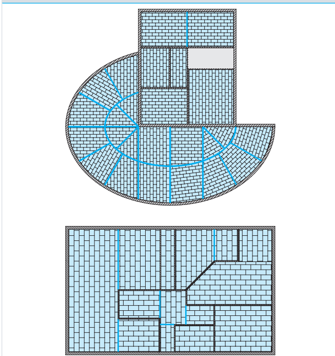
En las zonas de aberturas de puertas, reforzar la junta con pedestales
