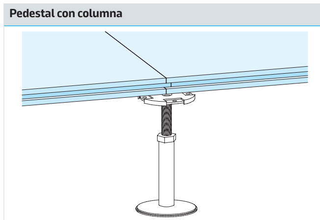
Pedestal con columna M16 para placa Tecnosol y Tecnosol Plus
