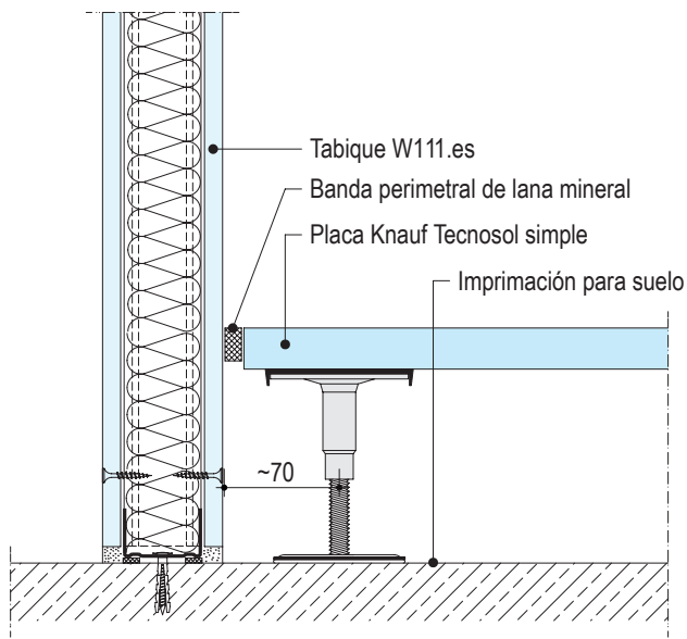
F181.es-V4 Montaje de instalaciones con pedestal bajo junta
