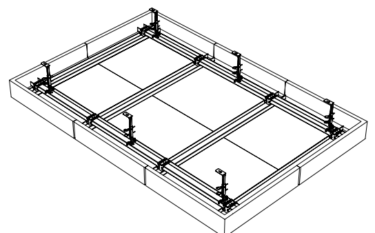
6) Стандартен елемент 1200
