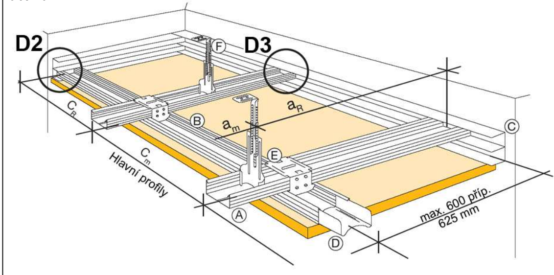
Maximální vzdálenost konstrukce pro třídu průhybu 1 podle EN 13964 (max. průhyb L/500)
