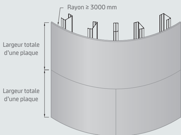
Disposition avec plaques entières, pour un rayon \geq 3000 mm
