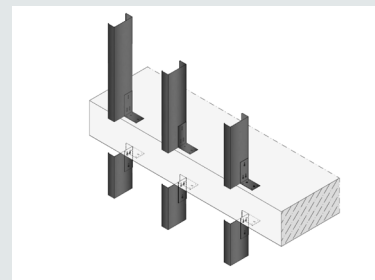
2. Installation de l'ossature extérieure à montants
