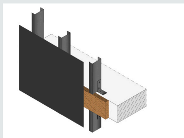
3. Isolation de l'extrémité des chapes et pose temporaire du pare-pluie sur les montants
