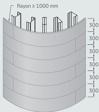
Disposition avec des bandes de 300 mm de large, pour un rayon \geq 1000 mm
